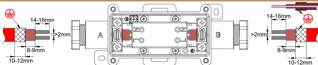
Modell mit zwei Heizkabeln (Y502)
